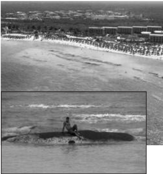
Fig. 7: Imagen de los geotubos paralelos a la playa donde se puede apreciar su tamaño
