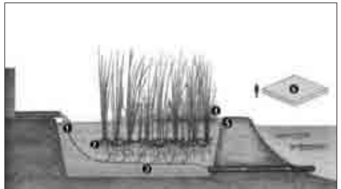
Humedal artificial de desechos cloacales e industriales
